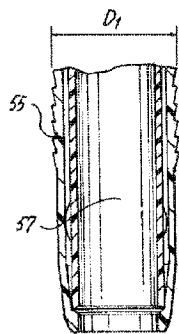
図10 (先行技術)
